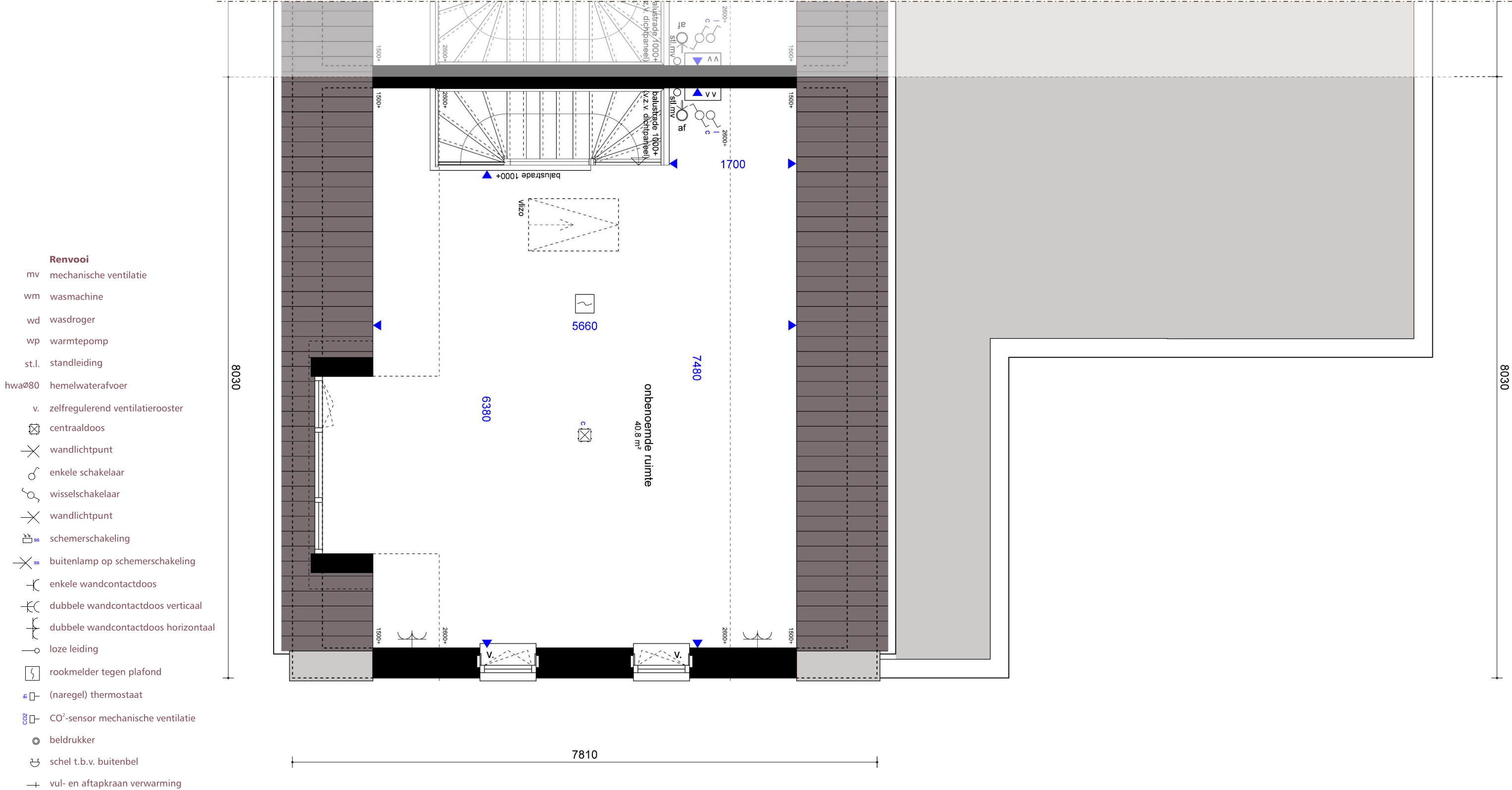
SCHAAL 1 OP 50 Plattegrond ~ Eerste verdieping
